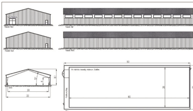
* Hallen skal ha ein innvendig aktivitetsflate på 20x60 meter, samt plass til kiosk og liten tribune. Seinare vil rideklubben sjå på moglegheita for å bygge på stallareal. (Skisse: Volda Rideklubb)
