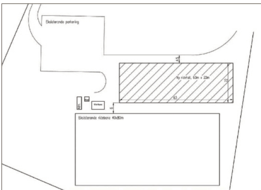
* Volda Rideklubb vil bygge ridehall ved sidan av der ridebana ligg i dag. Arealet vart opparbeidd då det vart nytta som riggområde under opprustinga av Botnavegen. (Skisse: Volda Rideklubb)
